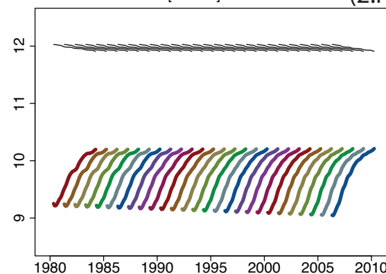
NSIDC SIE [10 6 km 2 ] (2.i)
