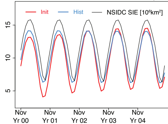
NSIDC SIE [10 6 km 2 ] (2.f)
