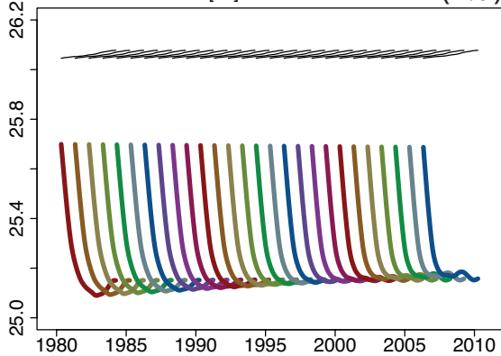
ERSSTv3b [°C] (2.g)
