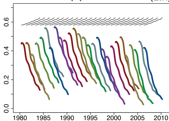
ERSSTv3b [°C] (2.h)
