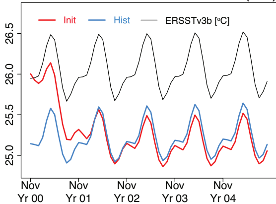
ERSSTv3b [°C] (2.d)
