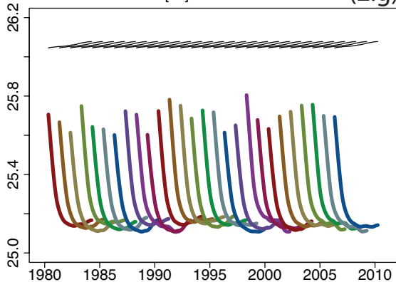
ERSSTv3b [°C] (2.g)
