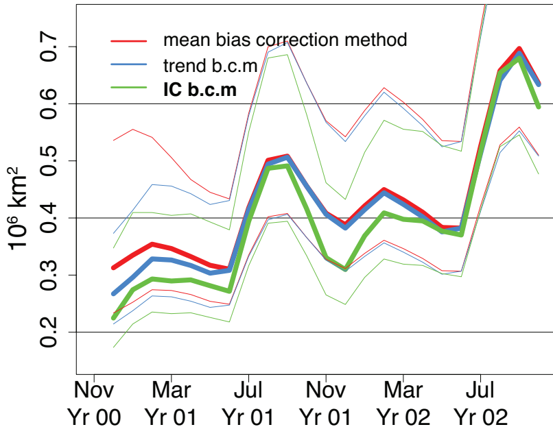
3-month smoothed RMSE of the NH sie
