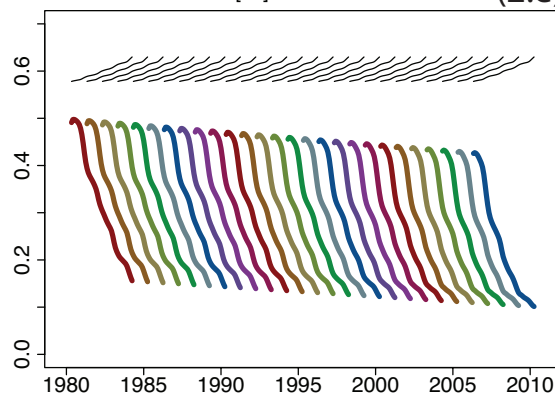
ERSSTv3b [°C] (2.h)
