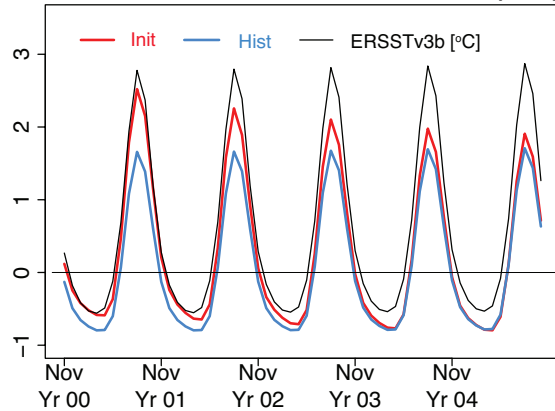
ERSSTv3b [°C] (2.e)
